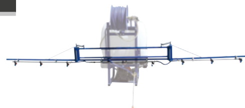
Spritzgestänge
