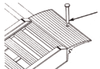
serienmäßige Bohrung in Auflagefläche für Abrutschsicherung mittels Bolzen
