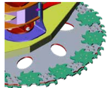
Mähscheibe Interpiquet High Cut mit auswechselbaren Messern
