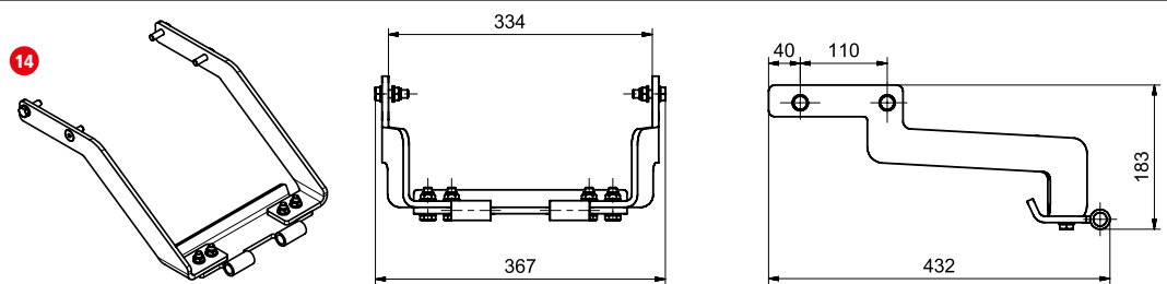
Adapter Efco, Silca, Alpine, 89 cm, 108 cm, Seco AJ, Snapper RPX Euro-Modelle
