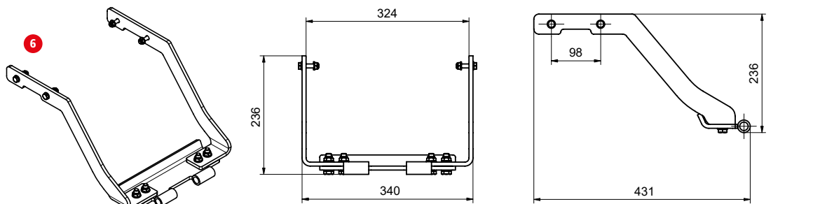
Adapter Castelgarden 92 cm, 102 cm „Großes Chassis“ NJ / TC Serie
